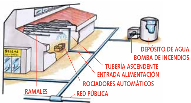
Sistema de rociadores automáticos.
