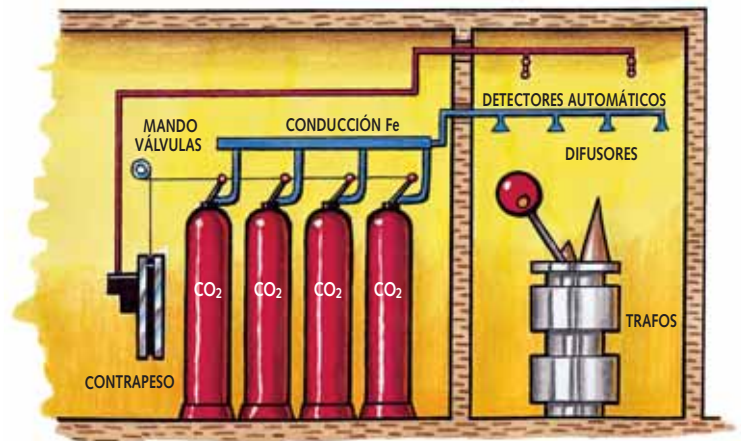
Sistema fijo de extinción por anhídrido carbónico.
